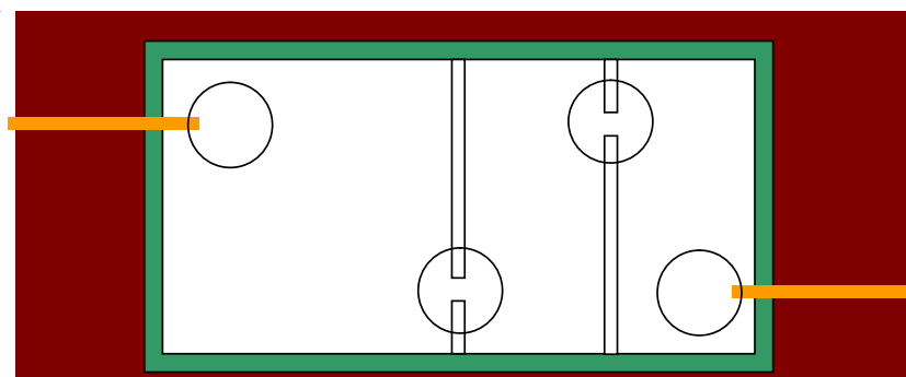
Mynd 4. Þriggja hólfa rotþrærtankur, séð ofanfrá
